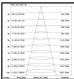
Répartition du flux lumineux
